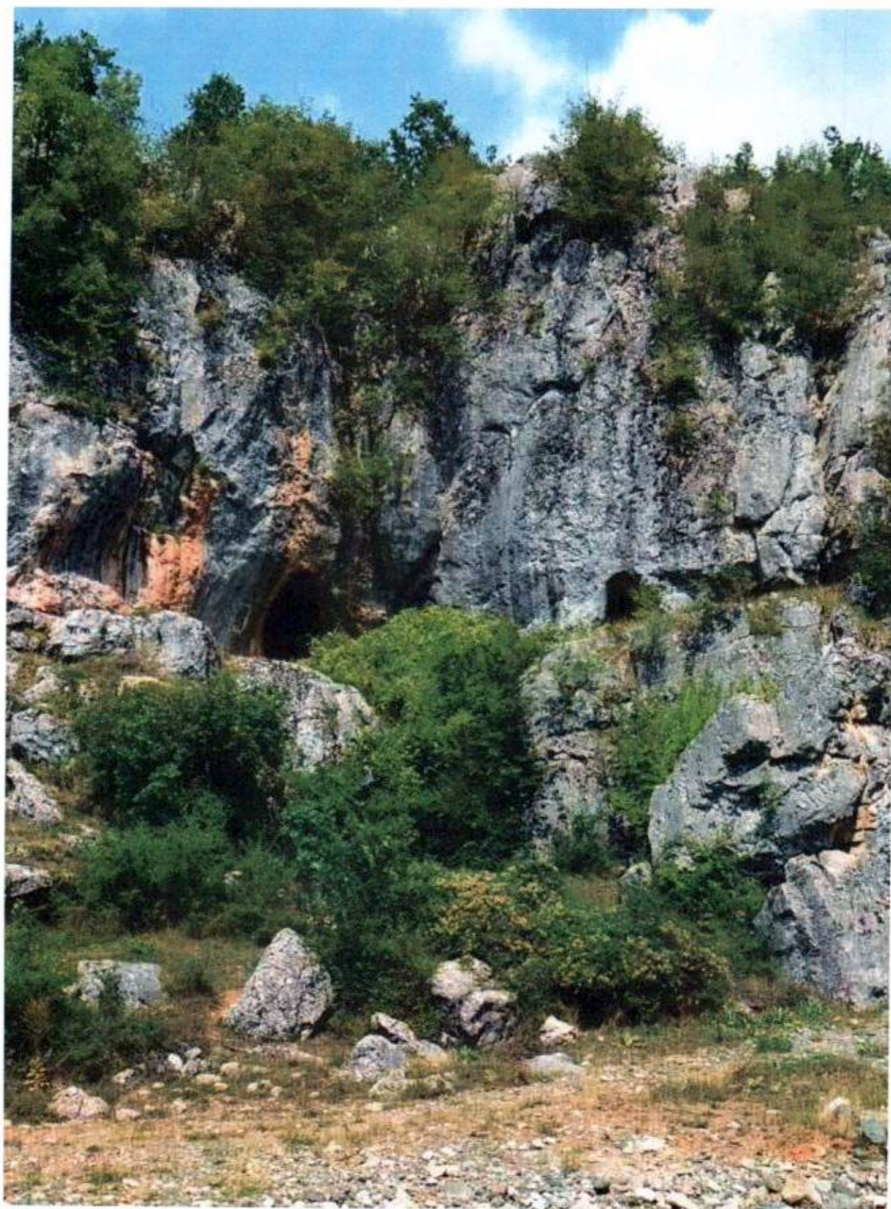
Figura 1.30 Pamje e jashtme e dy shpellave të Borovës, të cilat mendohen se kanë një lidhje mes tyre, për shkak të terrenit dhe përbërjes së shkëmbit ku ato gjenden.
